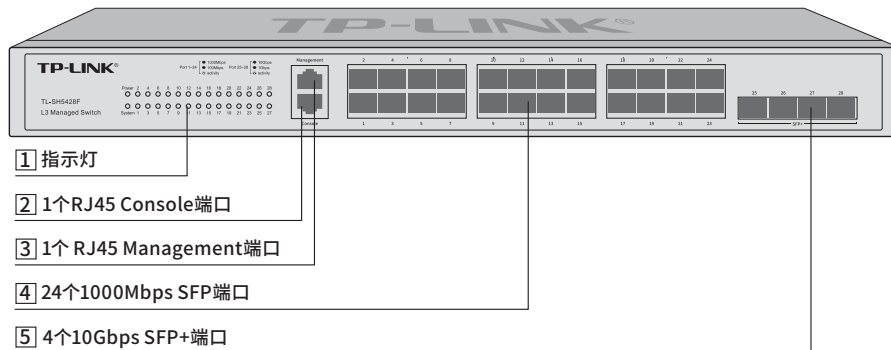
图1-4 TL-SH5428F前面板示意图
