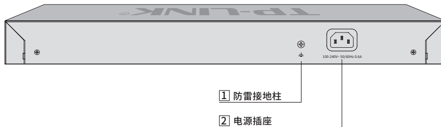
图1-9 后面板示意图
