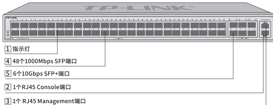
图1-5 TL-SH5654F前面板示意图
