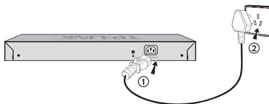
图3-5 电源线连接示意图
