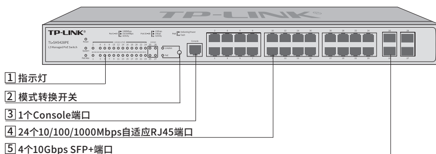
图1-8 TL-SH5428PE前面板示意图
