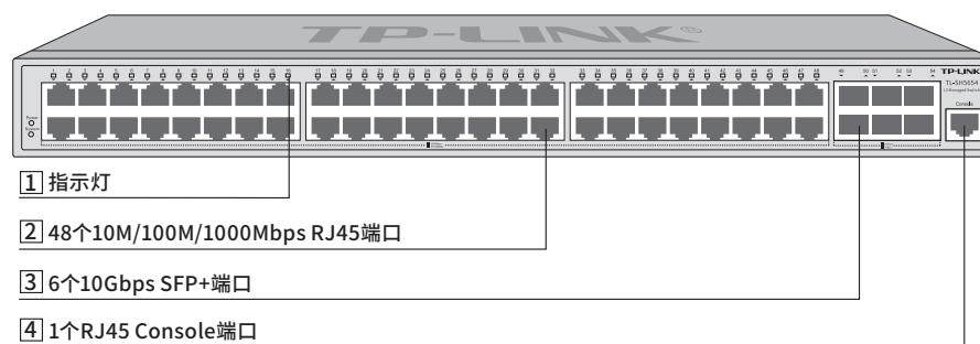
图1-2 TL-SH5654前面板示意图
