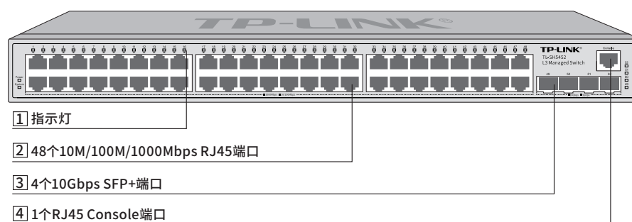
图1-3 TL-SH5452前面板示意图
