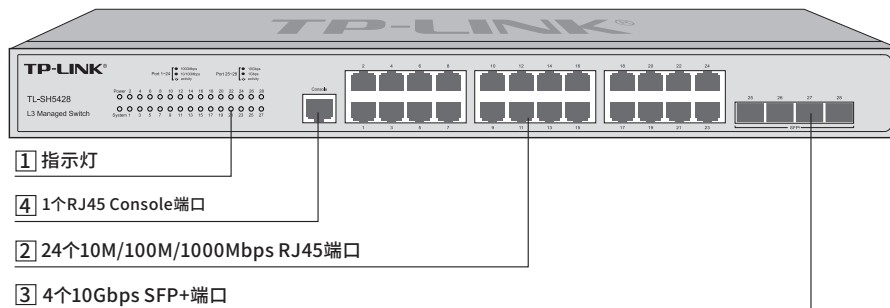
图1-1 TL-SH5428前面板示意图
