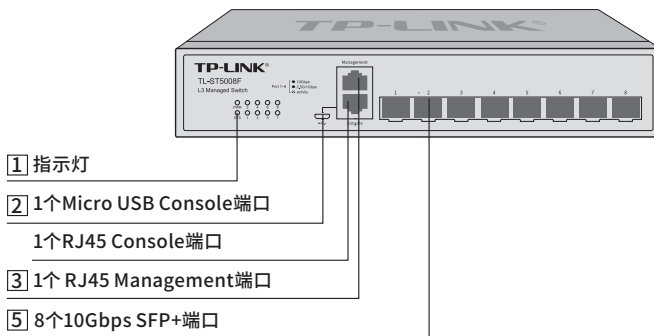
图1-6 TL-ST5008F前面板示意图
